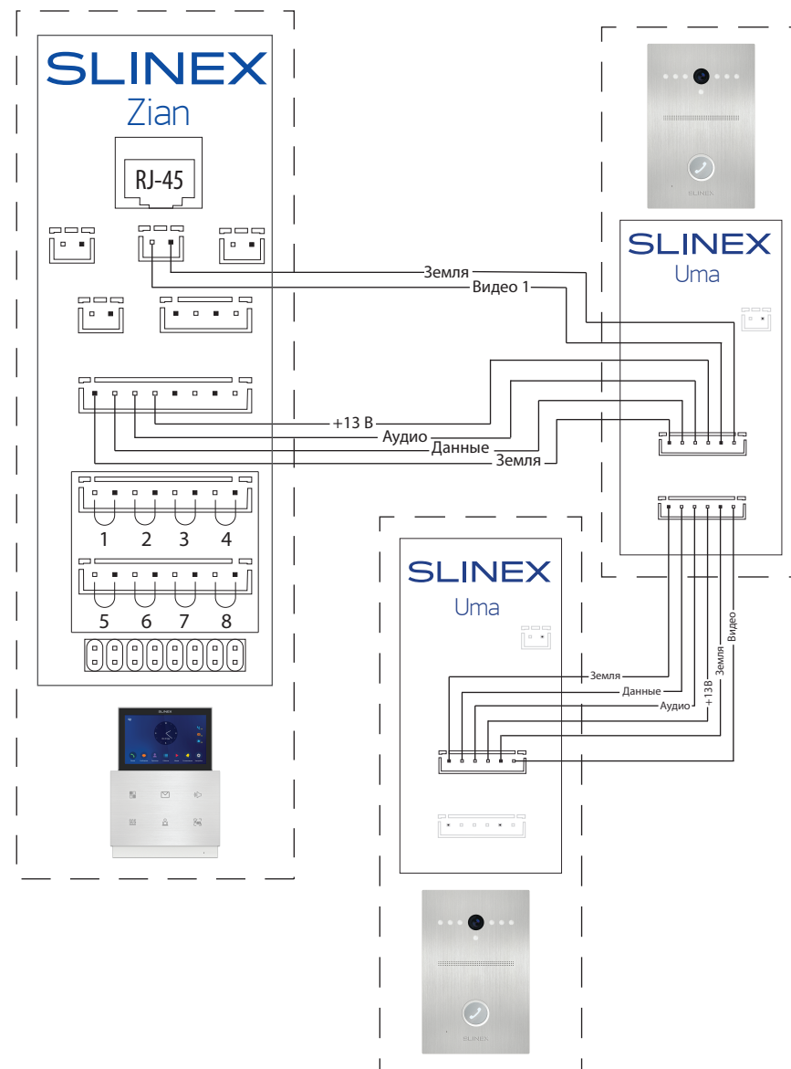
Схема 2. Подключение двух вызывных панелей.
