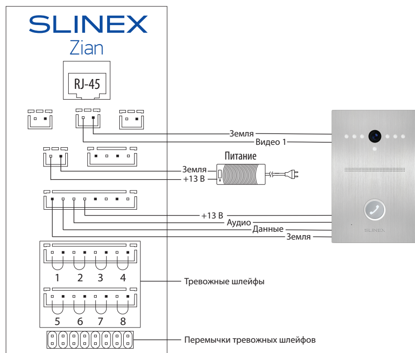
Схема 1. Подключение питания и вызывной панели.
