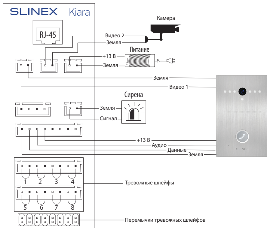
Схема 1. Подключение питания, вызывной панели, камеры и сирены.
