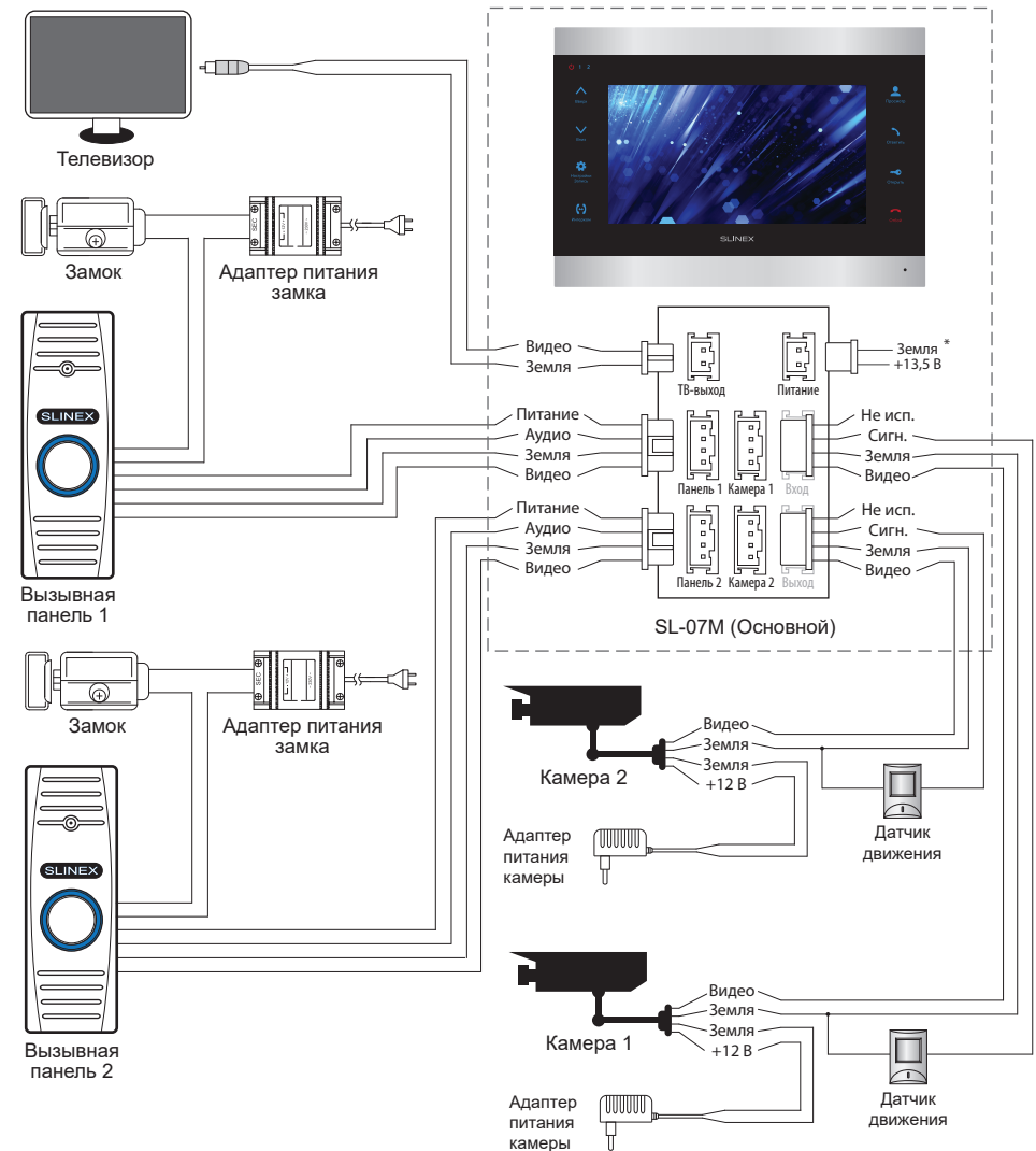
Схема 1. Подключение вызывных панелей, камер и телевизора к домофону SL-07M.
