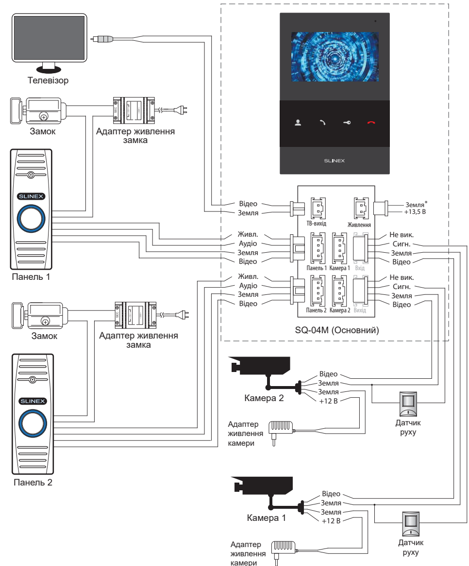
Схема 1. Підключення панелей виклику, камер і телевізора до домофона SQ-04M
