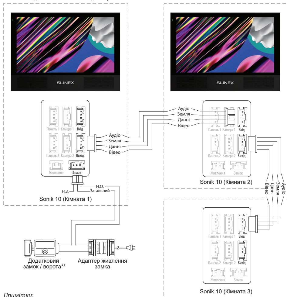
Схема 2. Підключення системи домофонів Sonik 10
